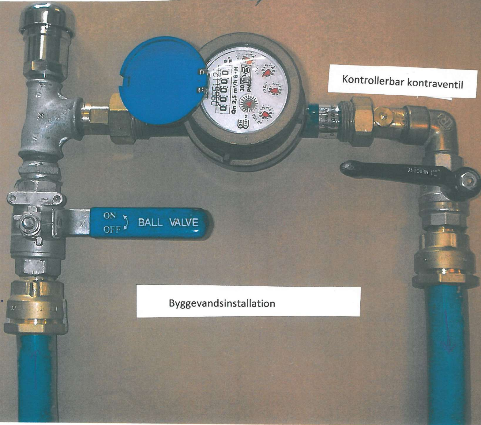
Rørafbryder med indbygget kontraventil
